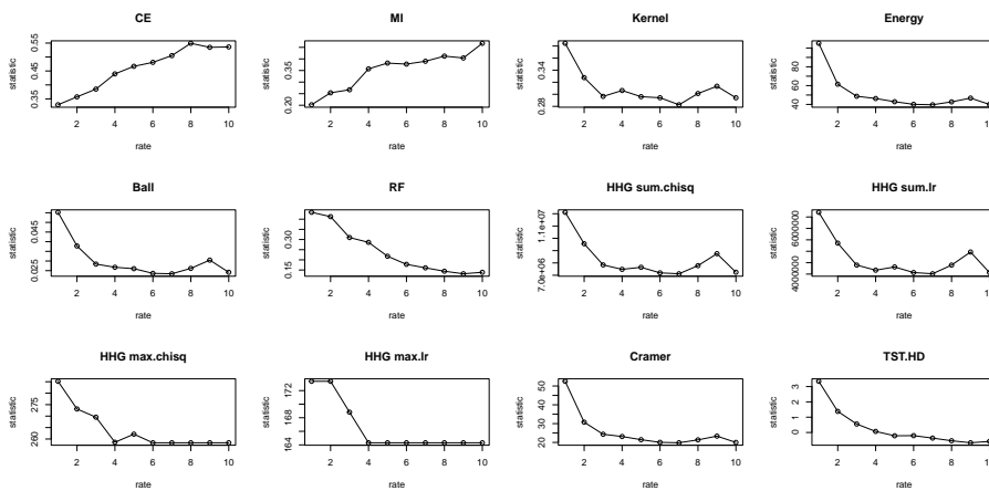
(c) 正态 copula 函数参数变化实验
